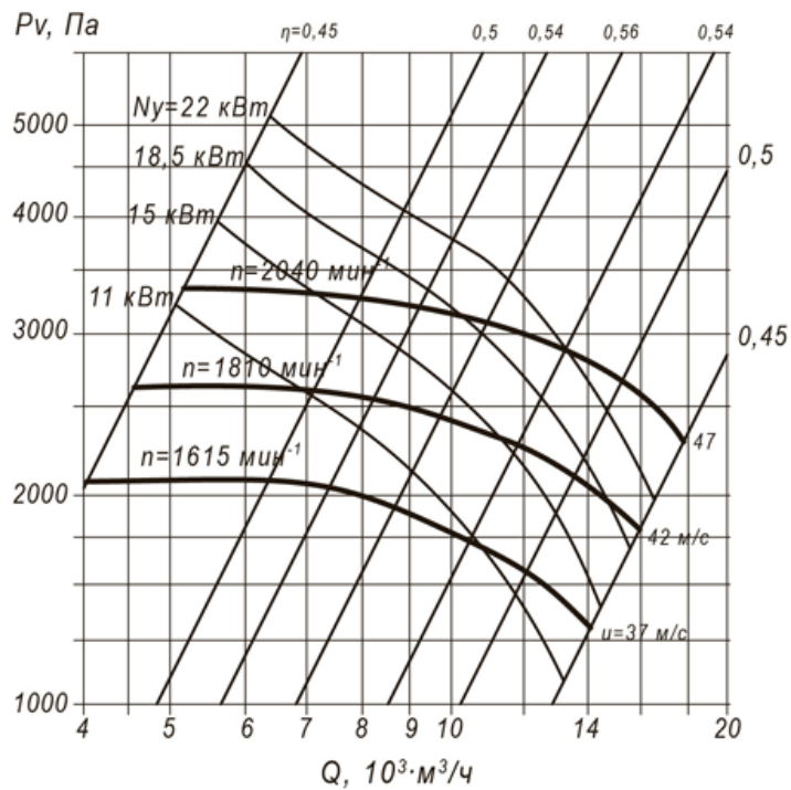
Аэродинамическая характеристика ВР 100-45 №6,3
