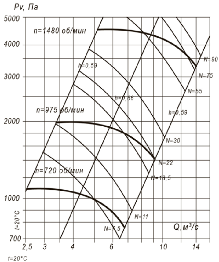
Аэродинамическая характеристика ВР 100-45 №10
