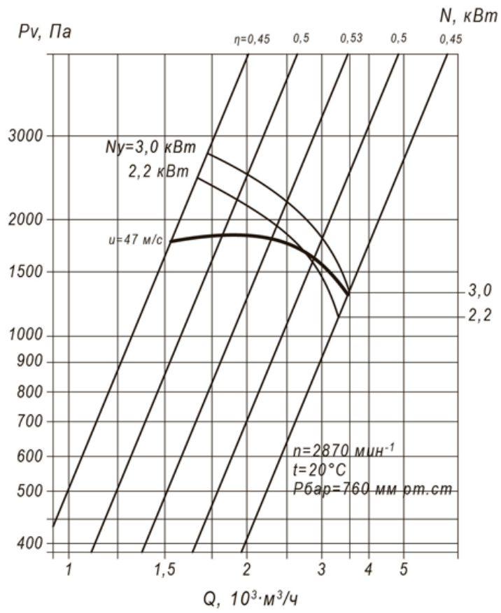
Аэродинамическая характеристика ВР 100-45 №4
