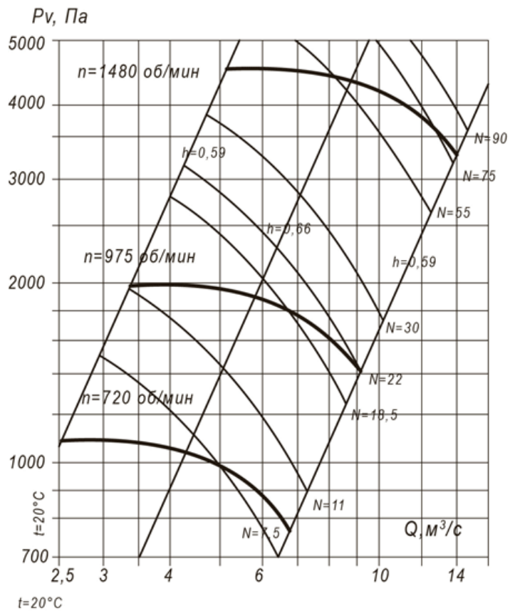
Аэродинамическая характеристика ВЦП 7-40 №10
