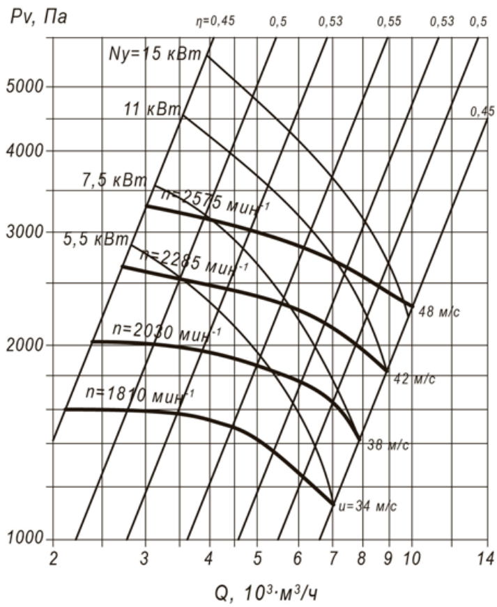
Аэродинамическая характеристика ВЦП 7-40 №6,3
