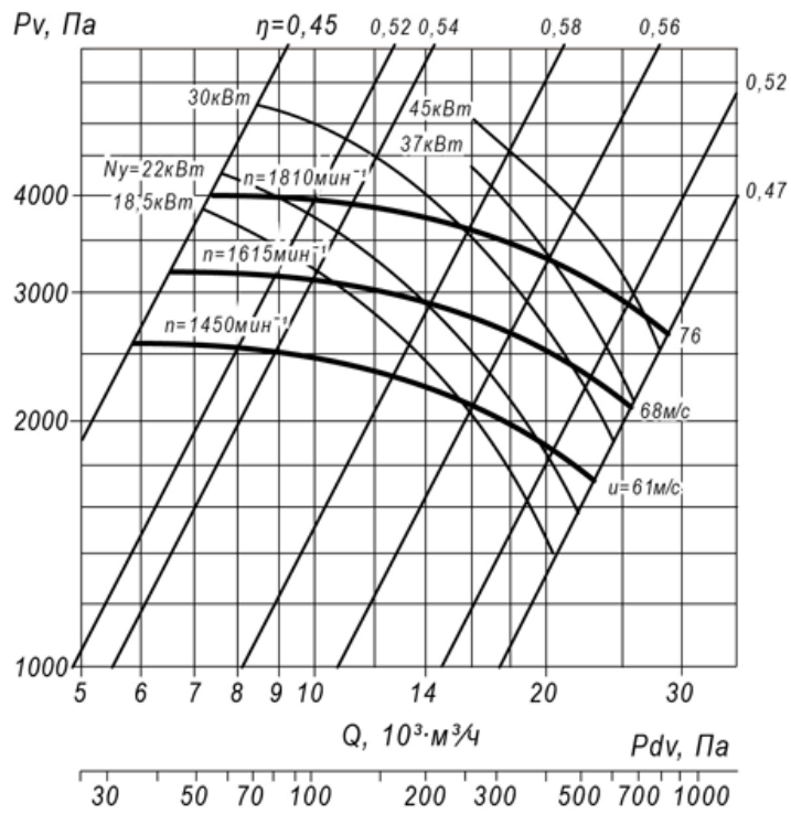
Аэродинамическая характеристика ВЦП 7-40 №10
