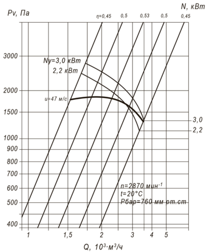
Аэродинамическая характеристика ВЦП 7-40 №4
